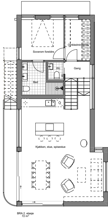
1:100 Plan 2
